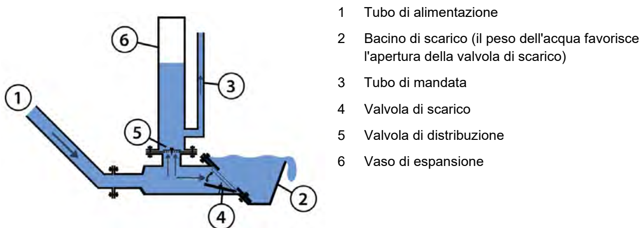
Figura 19: schema di una pompa ad ariete (fonte: ideozone.org).
